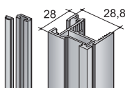
Profil S19
