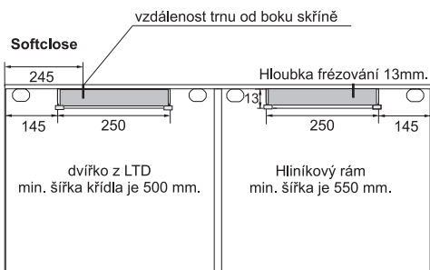
Profil S04N
