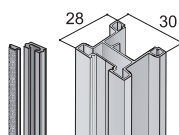
Profil S19
