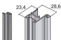
Profil S24
