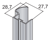
Profil S13B
