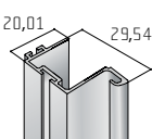
Profil S14
